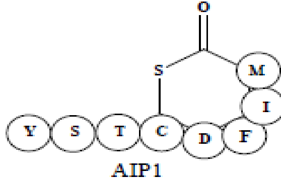
Şekil 3. AIP sinyal molekülünün yapısı (5)
