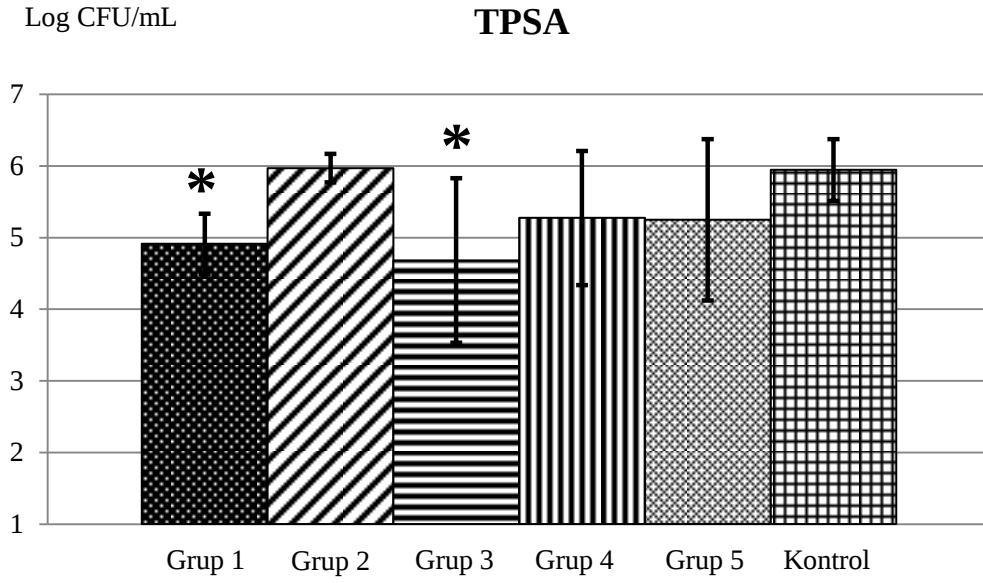
Şekil 24. Ön zenginleştirme sonrası QS inhibitörlü ve kontrol TPSA besiyerlerinde bireylerin ortalaması alınarak hesaplanan canlı hücre sayıları. (ortalama ± ortalamanın standart sapması, * p < 0.05 )
