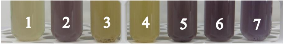
Resim 2. C. violaceum 'da viyolasin üretimi inhibisyonunun kalitatif olarak gösterilmesi (1, grup 1; 2, grup 2; 3, grup 3; 4, grup 4; 5, grup 5; 6, vanilin; 7, kontrol)
