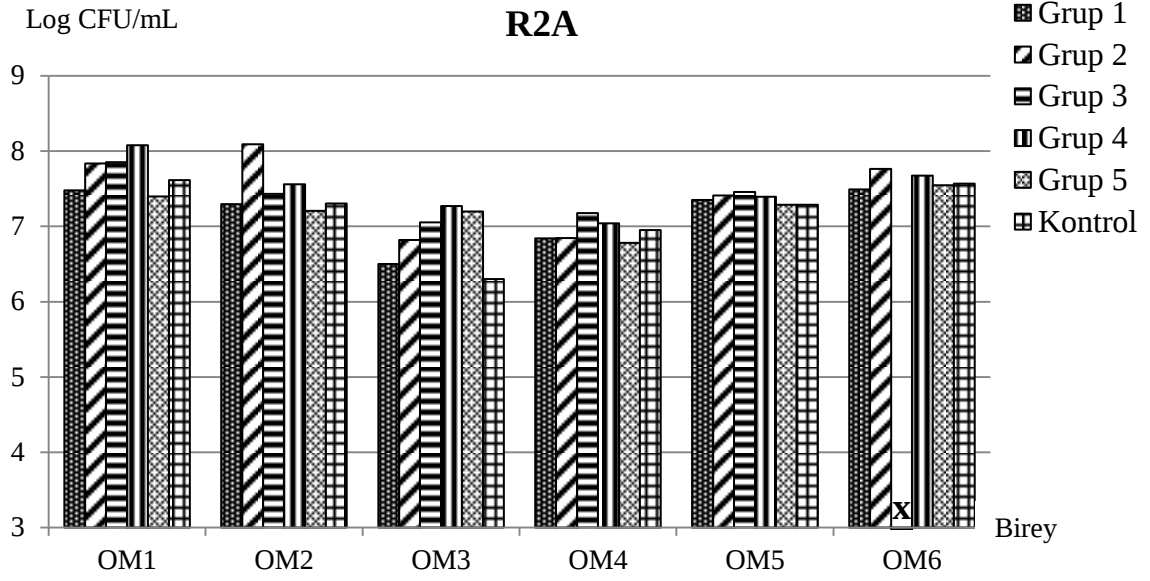
Şekil 16. QS inhibitörlü ve kontrol R2A besiyerlerinde izole olan canlı hücre sayıları (x: swarming tarzındaki üremelerden dolayı sayım yapılamadı)
