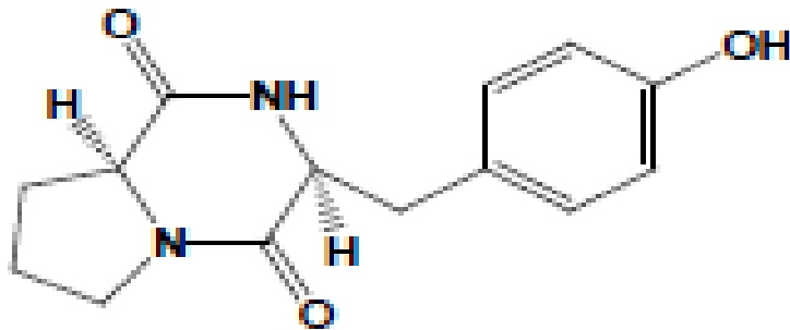
Şekil 4. Siklik dipeptit (L-Prolin-L-Tirozin) sinyal molekülünün yapısı (5)
