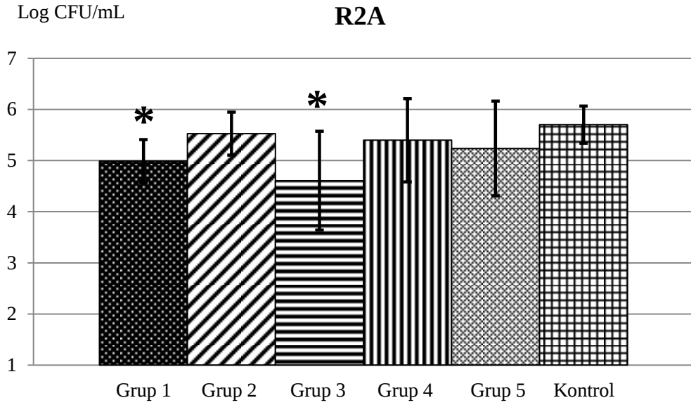
Şekil 25. Ön zenginleştirme sonrası QS inhibitörlü ve kontrol R2A besiyerlerinde bireylerin ortalaması alınarak hesaplanan canlı hücre sayıları. (ortalama ± ortalamanın standart sapması, * p < 0.05 )
