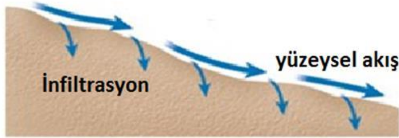
Şekil 9. Sıkışmaya uğrayan topraklarda yüzeysel akış-infiltrasyon ilişkisi
