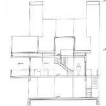
B-B Kesiti
