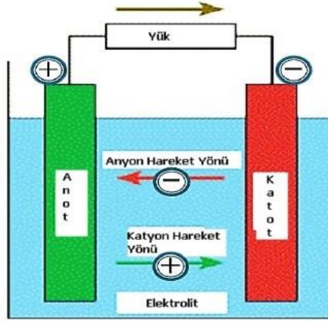
Şekil 1. Elektroliz hücresi (şematik)
