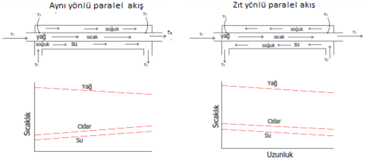
Şekil 4. Aynı yönlü ve zıt yönlü paralel akışlar için sıcaklıkların ısı eşanjörü boyunca değişimi
