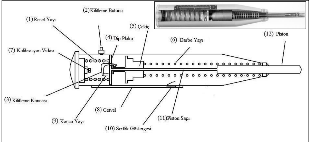
Şekil 1. Schmidt çekicinin genel kısımları
