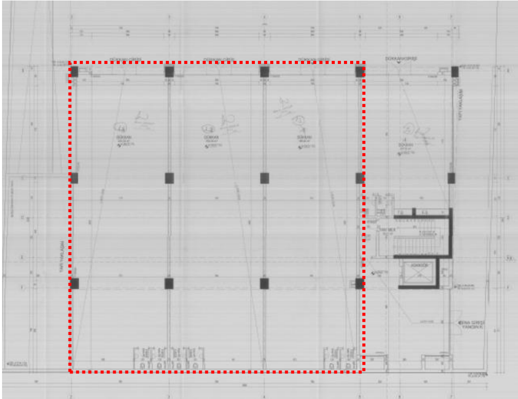
1. Bodrum Kat Planı (Mevcut Giriş Katı -4.00 kotu)
